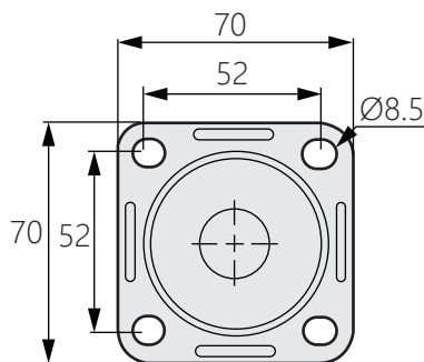
底板尺寸
