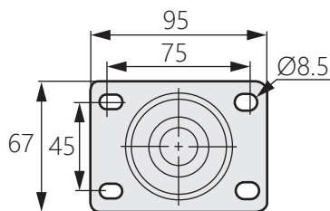
A3美式底板尺寸 2.5"
