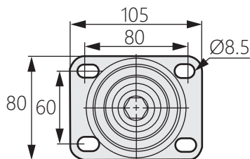
E4歐式底板尺寸 3"
