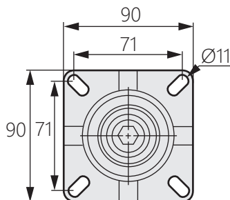
J5底板尺寸
