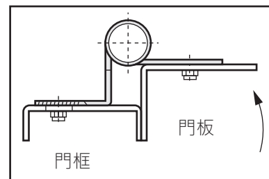
安裝示意圖
