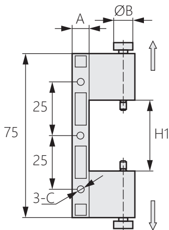
安裝圖
