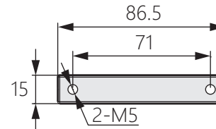
開孔尺寸
