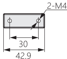
開孔尺寸
