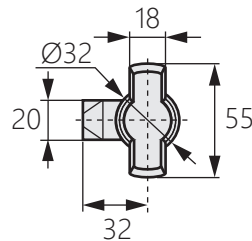
[ TM-1002-2 ] 無鎖
