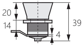
[ TM-1002-1 ] 有鎖
