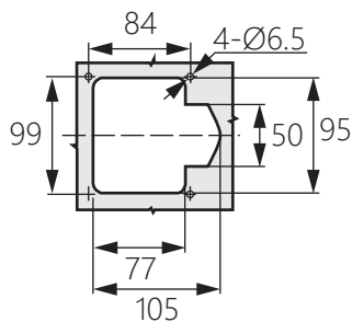
安裝開孔尺寸
