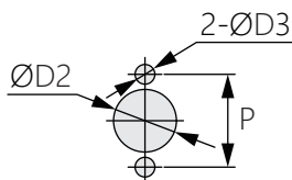
面板鑽孔尺寸
