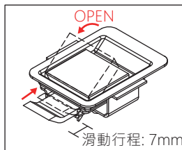
安裝示意圖
