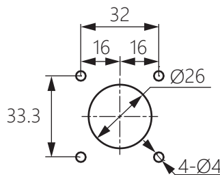
開孔尺寸
